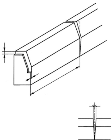
Rysunek 2 - Przykład kształtu przeznaczonego do ryglowania; wymagania dotyczące wymiarów i dopuszczalnych odchylek
