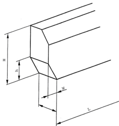
Rysunek 2 - Przykład kształtu przeznaczonego do ryglowania; wymagania dotyczące wymiarów i dopuszczalnych odchylek
